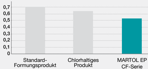
Vierkugel-Verschleißtest (ASTM D 4172*)
